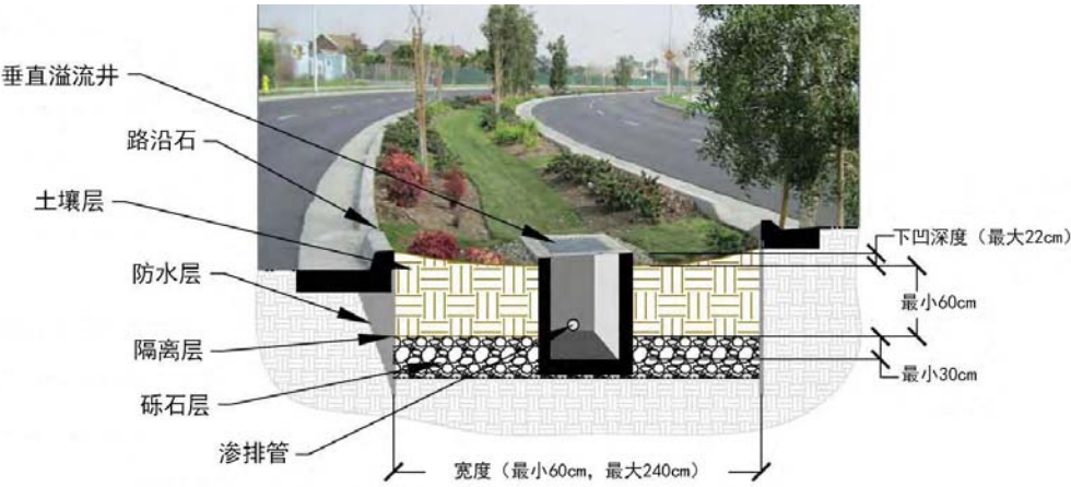
图 7-27 植草沟典型构造示意图
