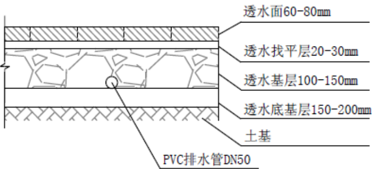
图 7-17 透水铺装构造示意图
