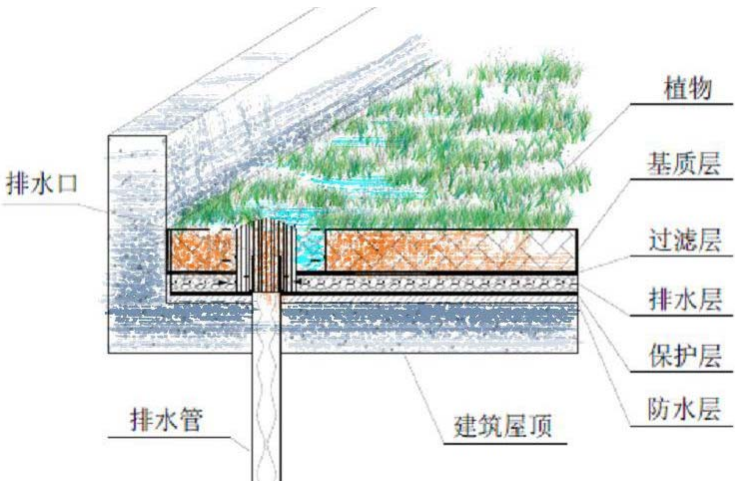
图 7-19 绿色屋顶典型构造示意图
