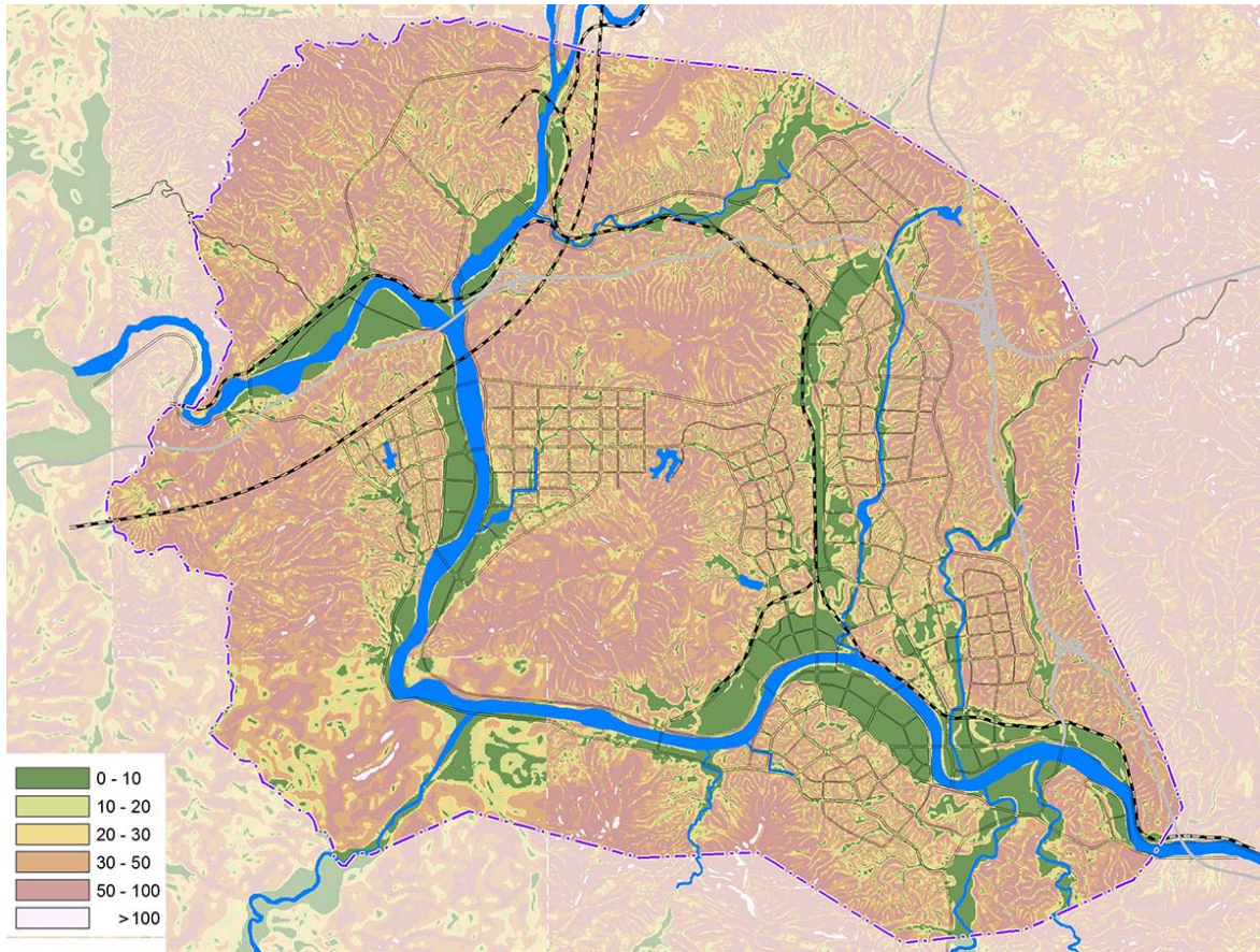
图 4-2 规划区坡度分析图
