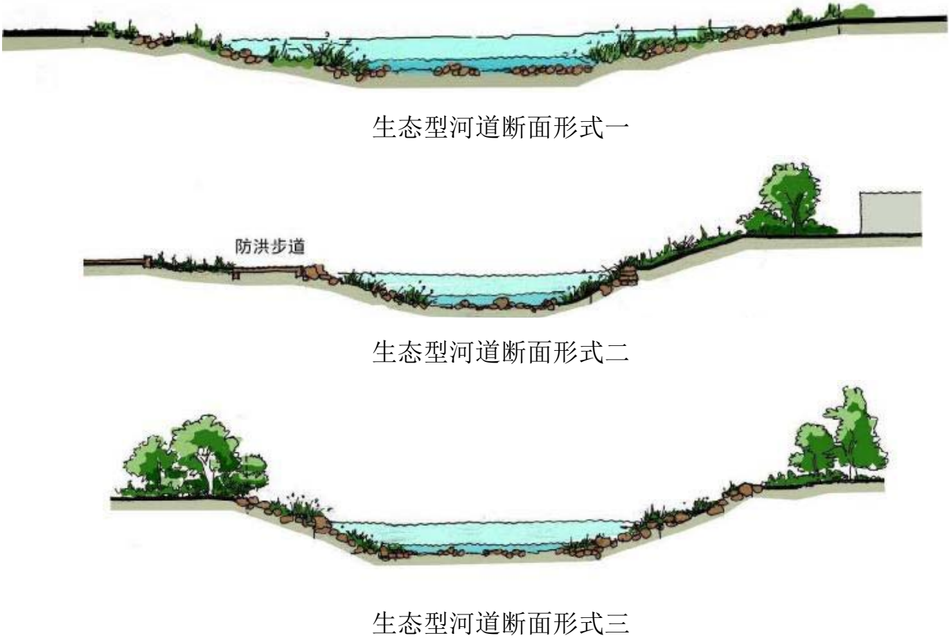
图 5-2 不同类型生态型河道断面驳岸改造示意图
