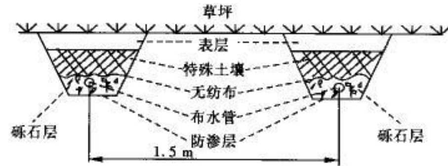
图 7-42 人工土壤渗滤典型构造示意图
