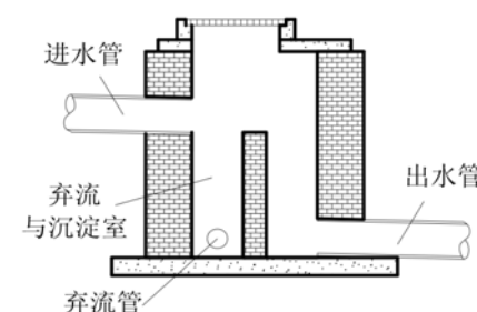
图 7-40 小管弃流井示意图
