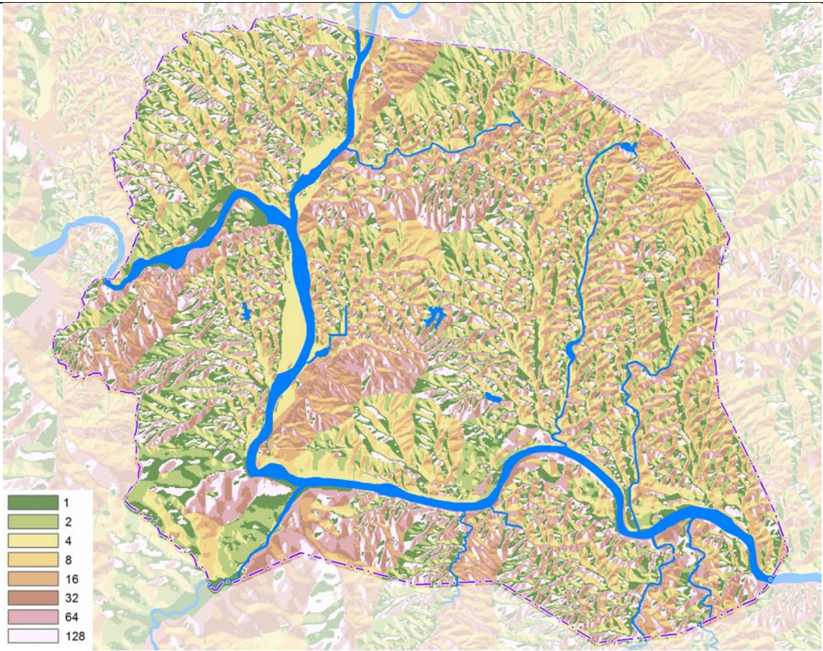
图 4-3 规划区汇流方向分析图
