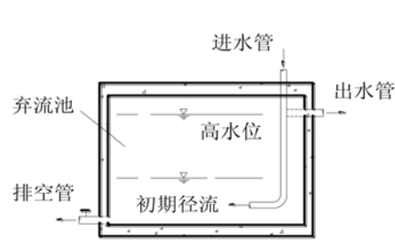
图 7-41 容积法弃流装置示意图
