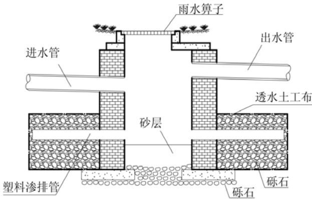
图 7-35 辐射渗井典型构造示意图
