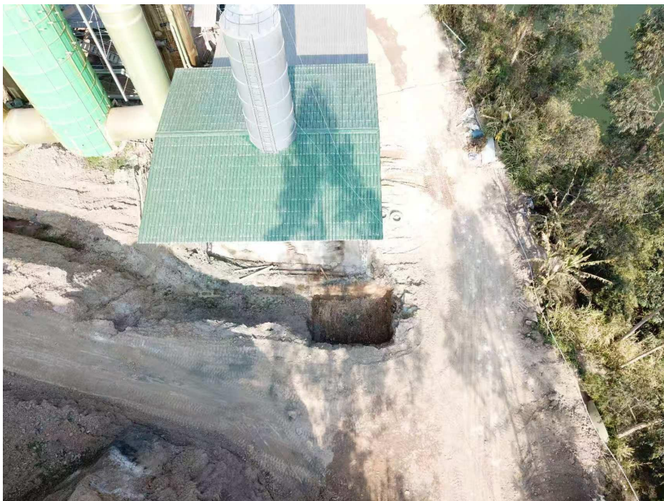
南侧截排水沟及沉砂池
